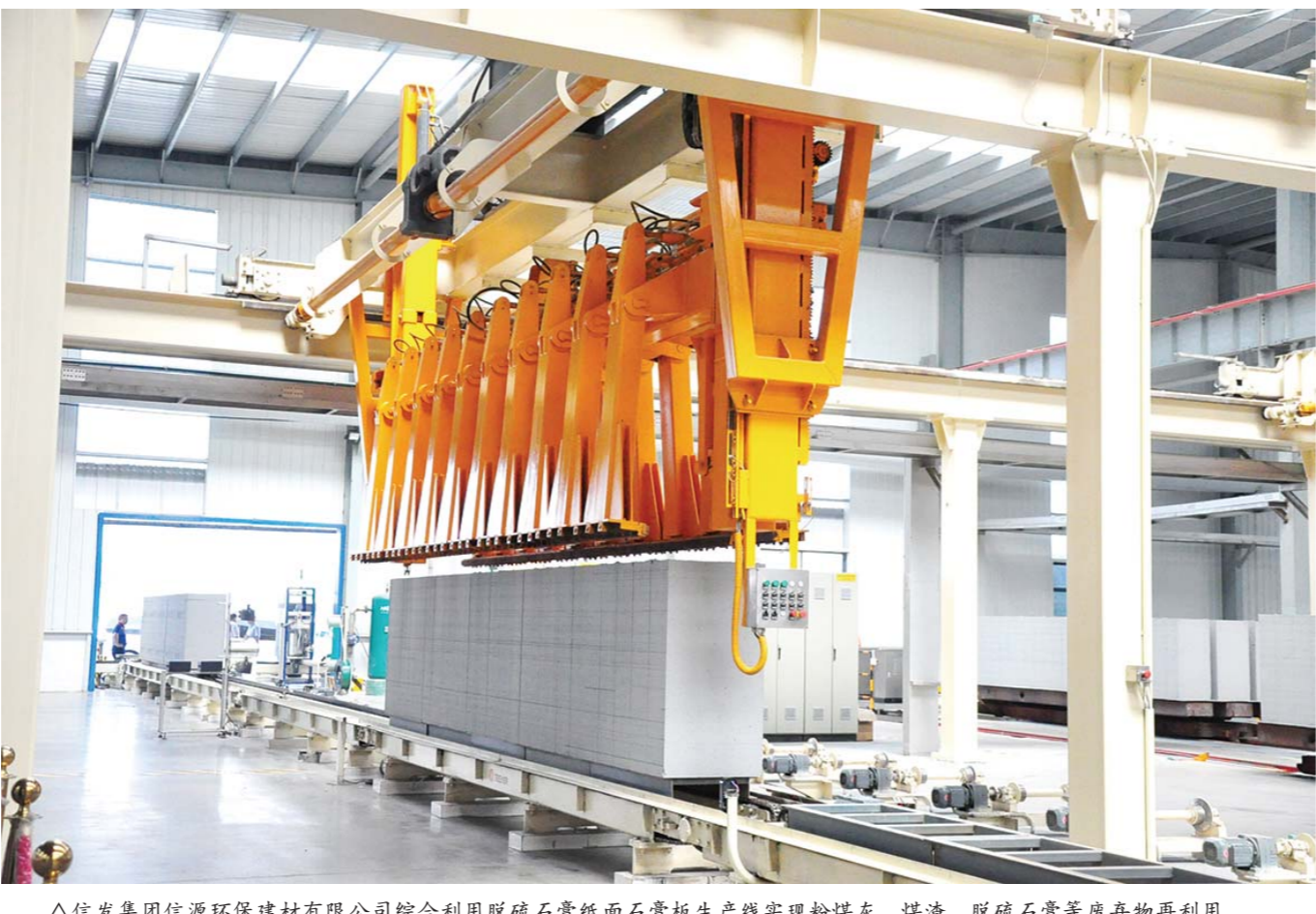
信发集团信源环保建材有限公司综合利用脱硫石膏纸面石膏板生产线实现粉煤灰、煤渣、脱硫石膏等废弃物再利用
