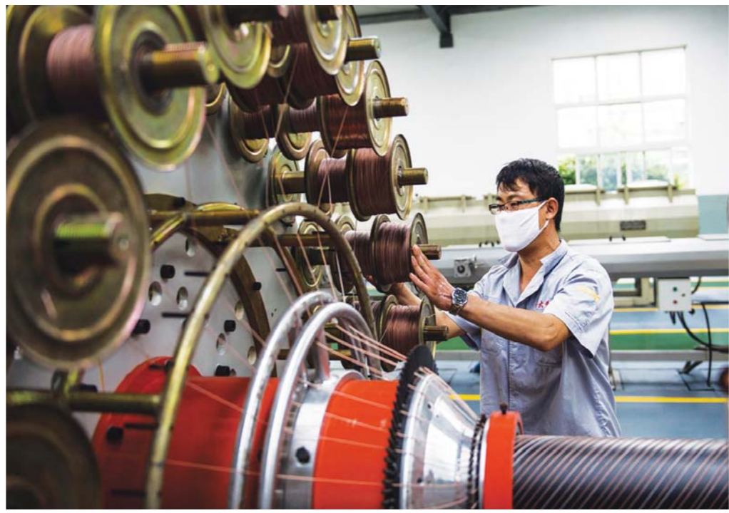
方大新材料公司工作人员检查钢丝网管架塑料复合管丝网。 (资料片)
