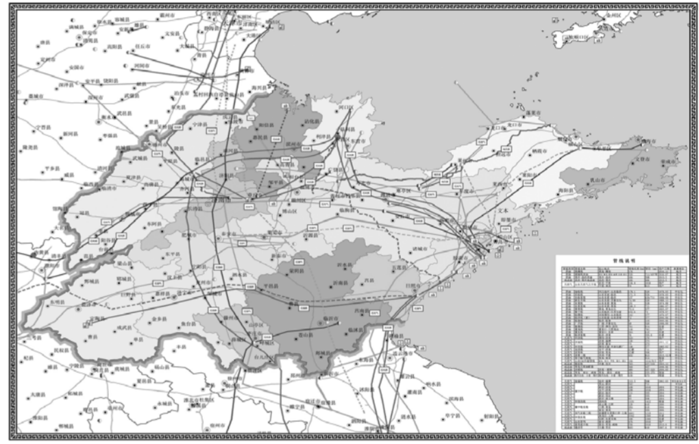
山东省境内油气管道走向示意图
