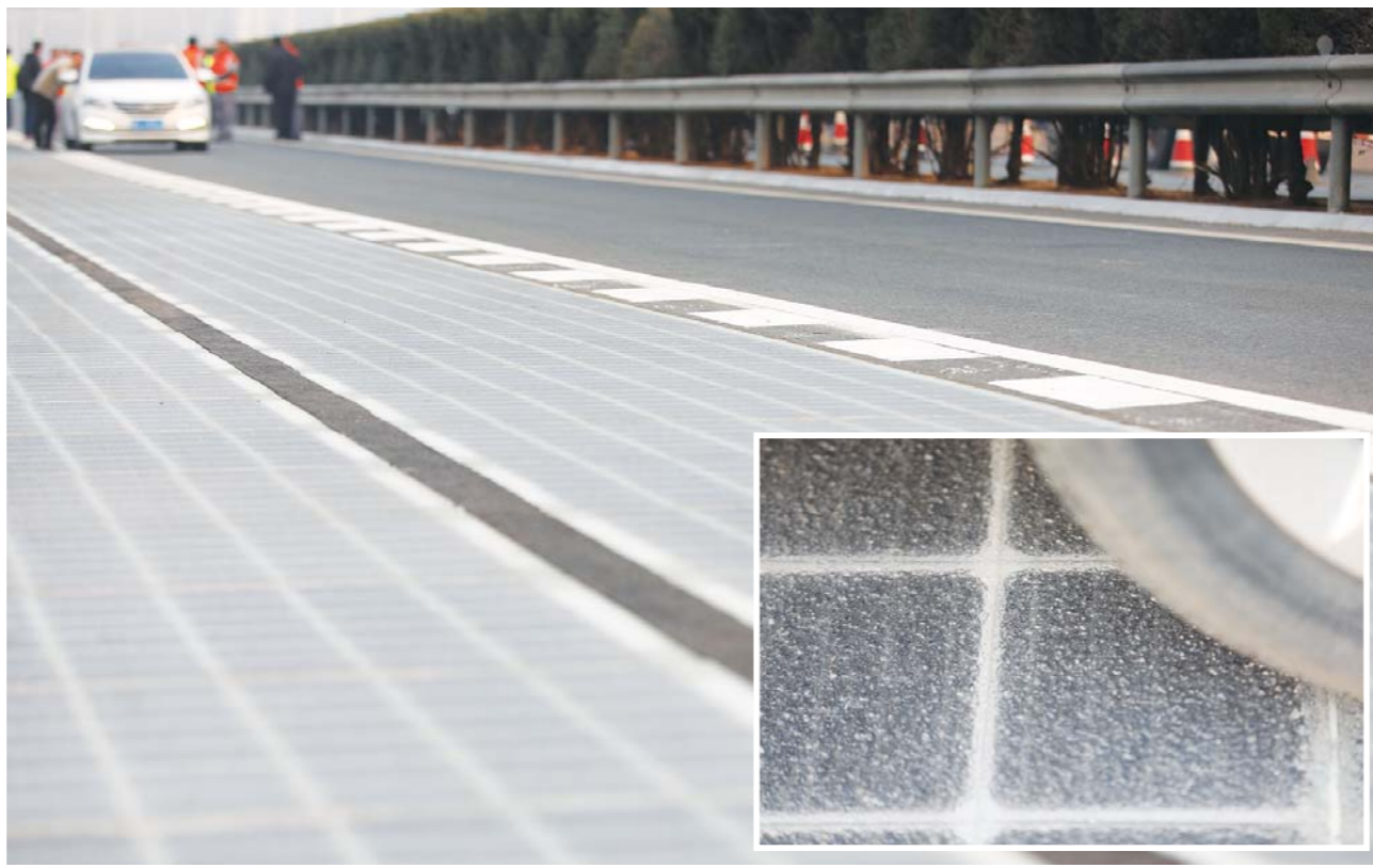
该试验段采用承载式光伏路面技术，将符合车辆通行条件的光伏发电组件直接铺设在高速公路路面上，从而实现太阳能发电。其承重能力、抗滑性能等路用性能指标均满足国家相关标准，可满足所有车型通行。
