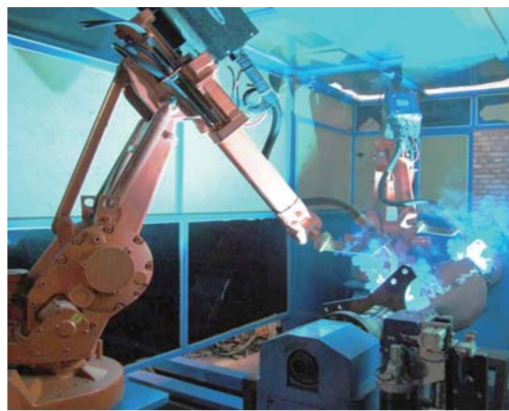
△“新三板”挂牌上市企业云宇制动器的机器人焊接生产线
