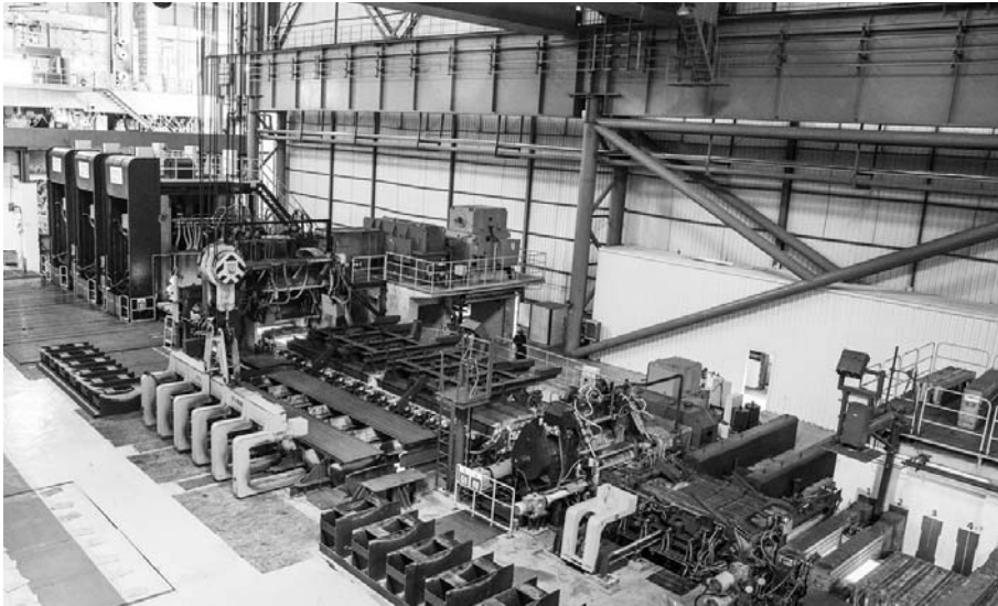
日钢ESP生产线现场。
