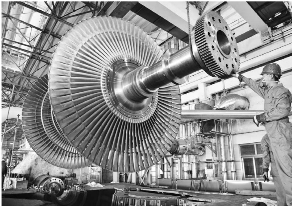
华能黄台电厂8号机组进行供热升级改造。(资料片)
