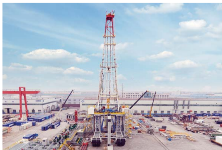
△石油装备3000HP智能一体化超深井快移钻机
