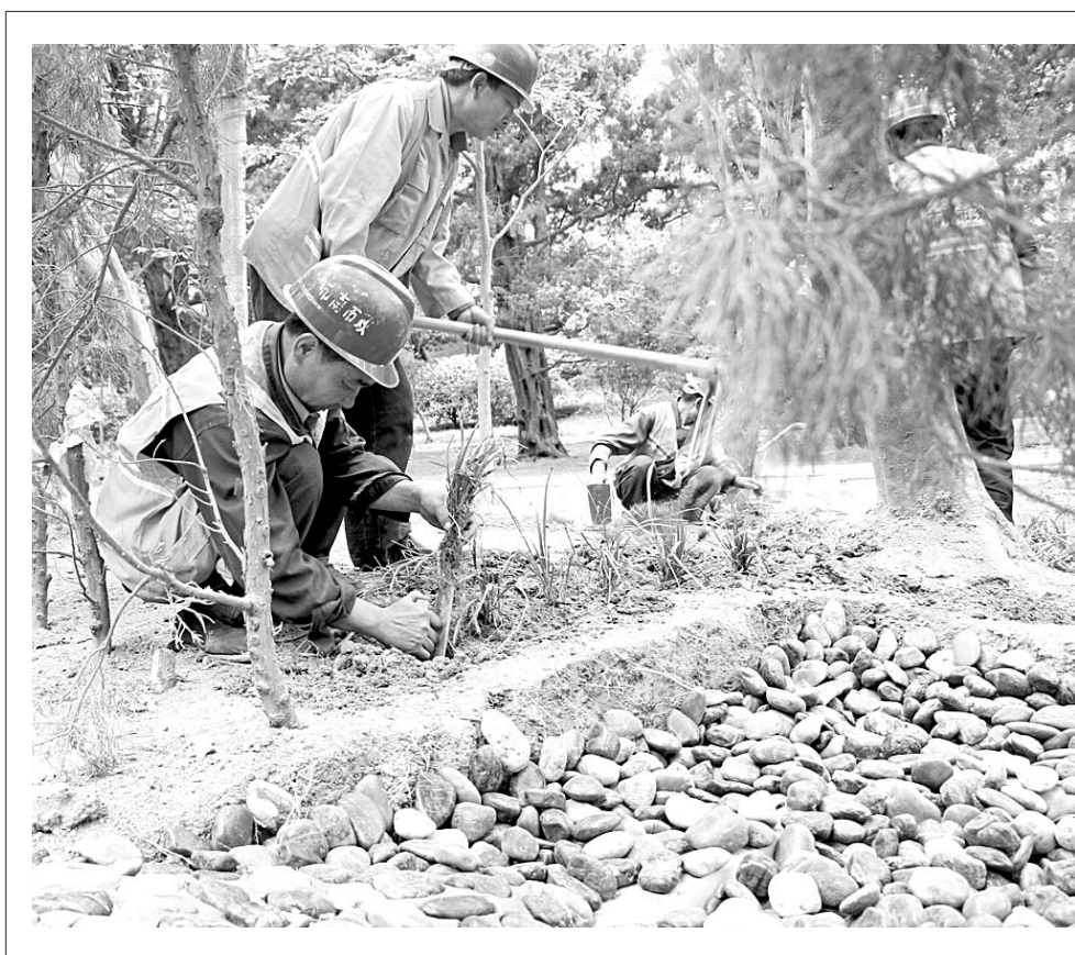
道路改造 引入“海绵”元素 □记者 薄克国 报道 6月13日，地处八大区域的临淮关路改造正在有序推进。 路段原存在网裂、碎裂等病害，为消除道路病害，市南区将该路段列入今年养护维修范围，同时结合道路周边条件，引入海绵元素对道路进行试点整治。作为青岛市首条海绵城市元素示范整治道路，改造后的临淮关路未设置市政排水管线，而是利用“渗、滞、蓄、净、用、排”建设理念，实现雨水的自然收集、散排。
