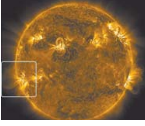
这是一张生成于2011年3月8日的太阳像。巨大“磁绳”就是发现于白色方框内的活动区。中美研究人员日前合作发现,太阳活动区存在着巨大“磁绳”,这种“磁绳”可能正是引发太阳风暴的罪魁祸首。
